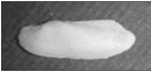
Barbartia angusta - 20 mm
