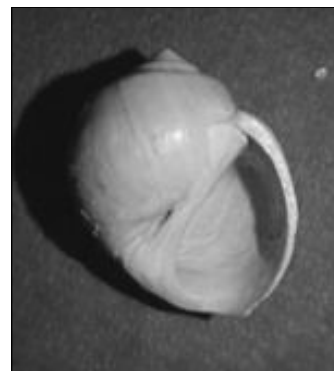
Ampullina parisiensis 25 mm
