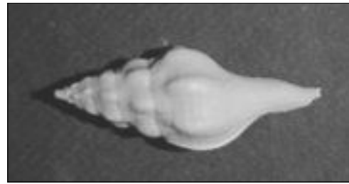
Clavilithes laevigatus - 32 mm
