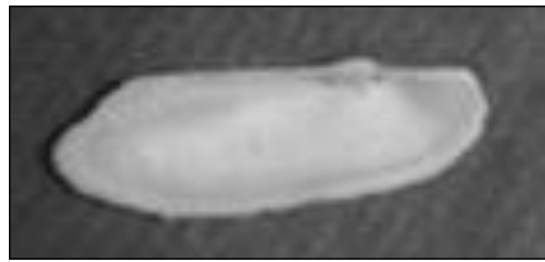
Barbartia angusta - 20 mm
